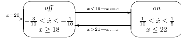
Fig. 1. Thermostat.
